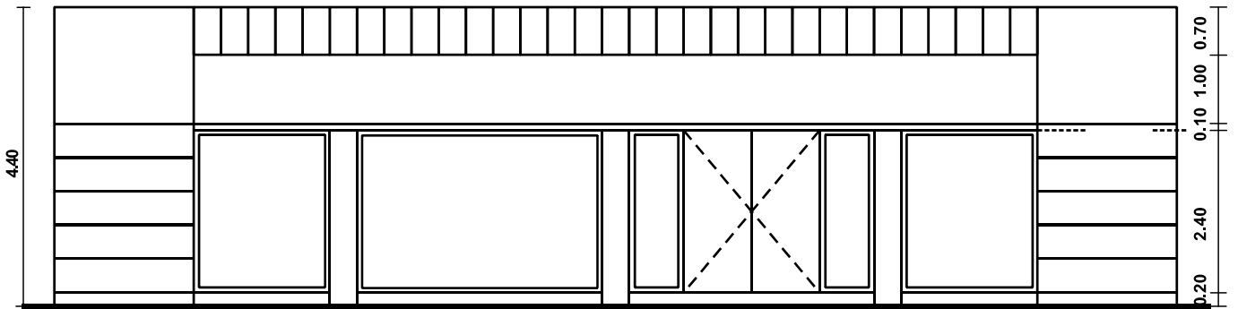
ΠΡΟΣΟΨΗ
