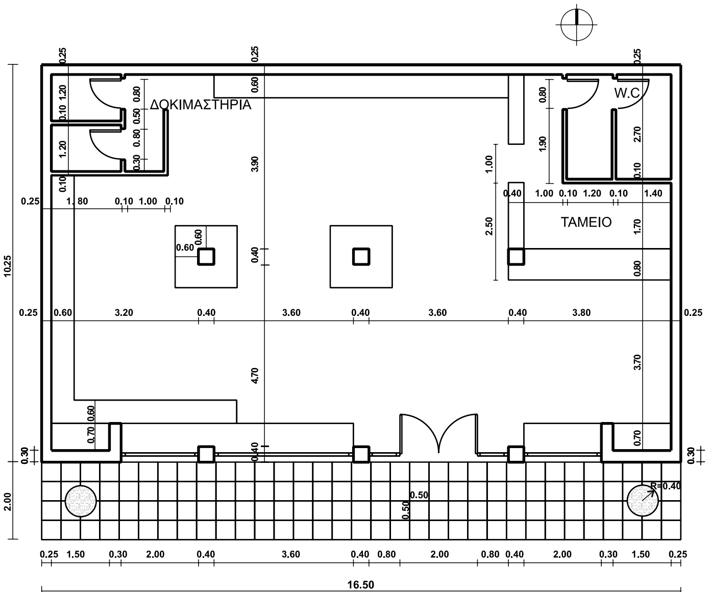
ΚΑΤΟΨΗ
